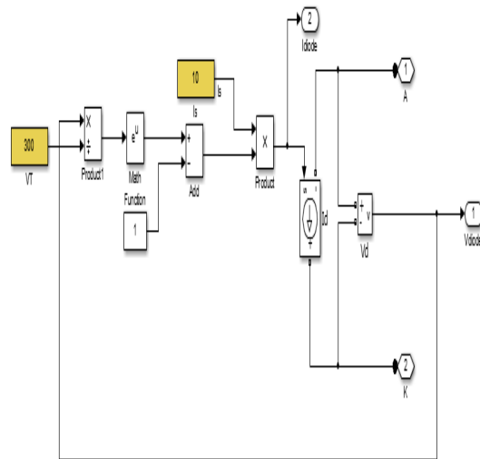
Fig. 11. PV Array Diode
